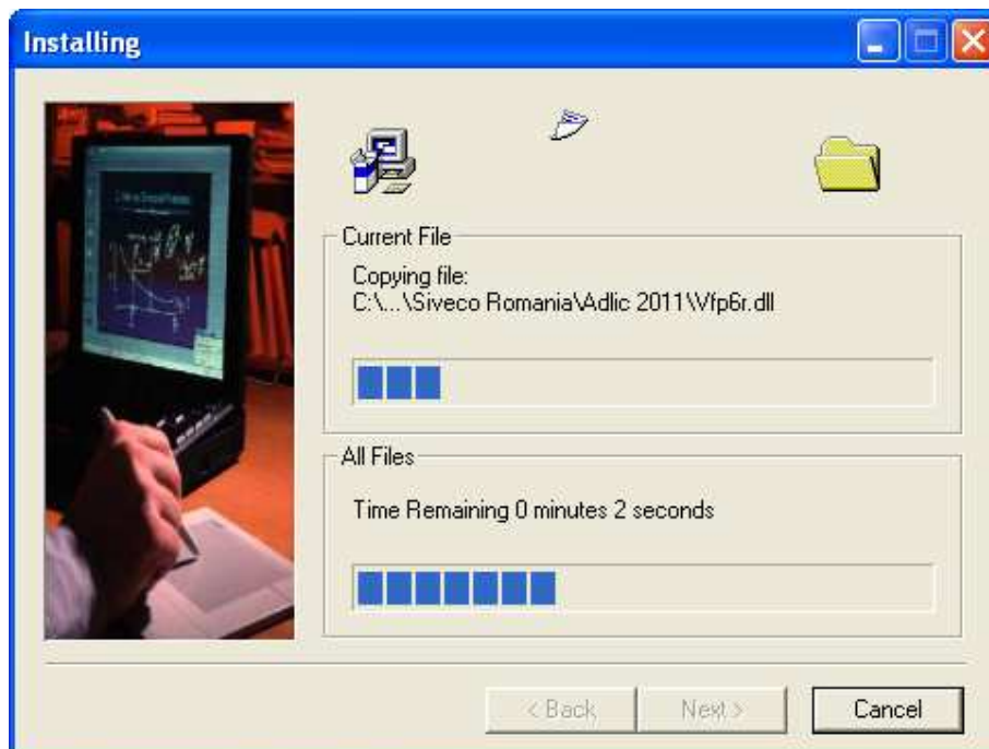
Figura 5. Instalarea aplicației
