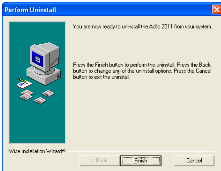
Figura 7. Confirmare dezinstalare
