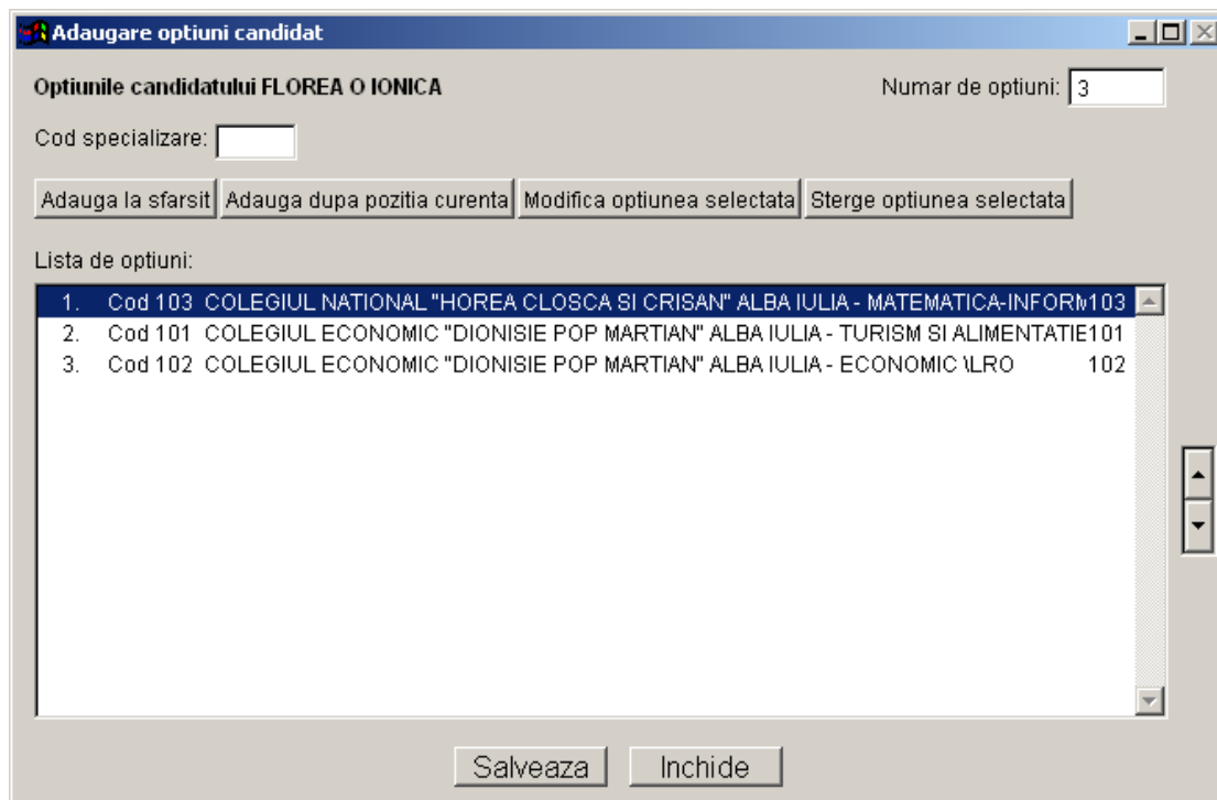
Figura 7 Adăugare opțiuni
