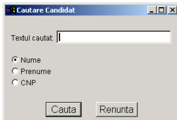
Figura 11 Caută candidat
